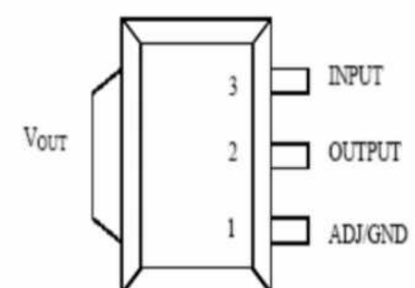
SOT89-3
